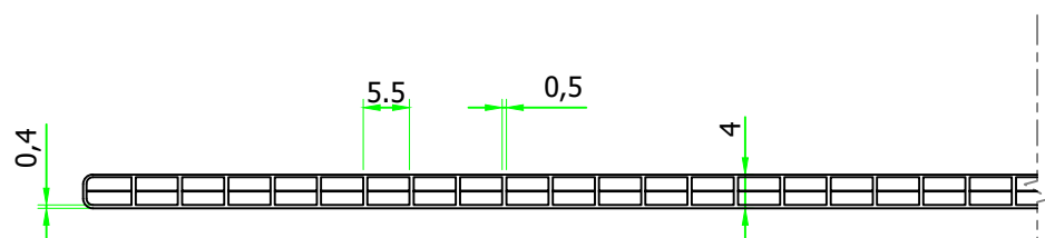
DETALLE LADO A ESCALA 1:1
