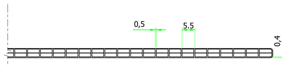
DETALLE LADO B ESCALA 1:1
