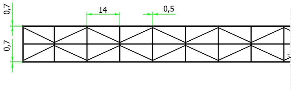
DETALLE LADO A ESCALA 1:1
